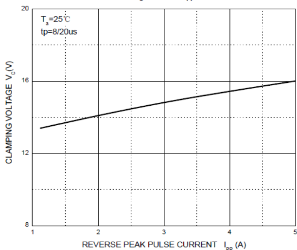
V_C — I_{PP}
