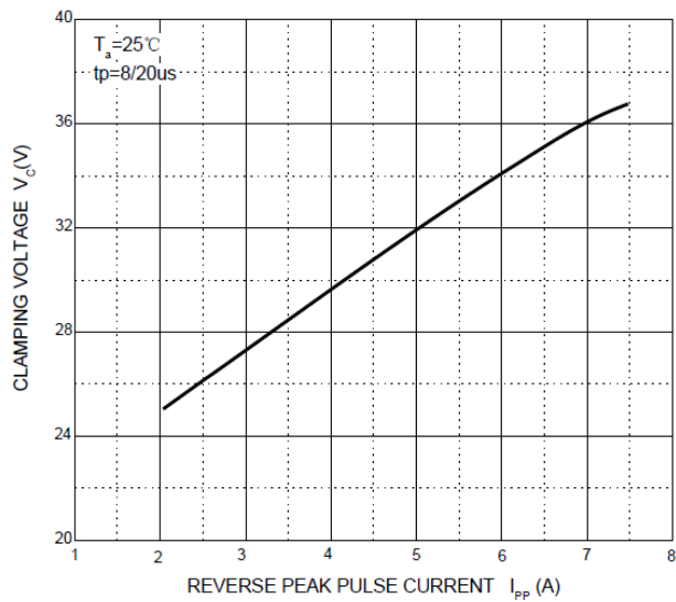
V_C — I_{pp}
