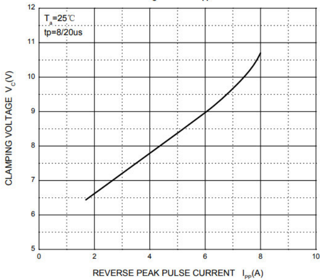
V_C — I_{PP}
